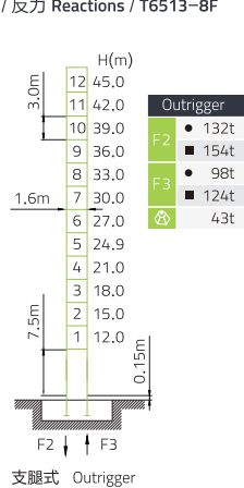
支腿式 Outrigger
