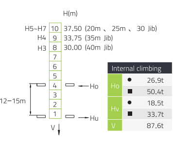
D25 内爬式 Internal climbing
