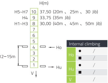
C25 内爬式 Internal climbing
