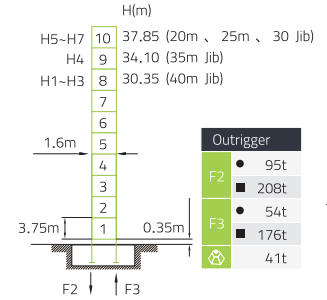
D25 支腿固定式 Outrigger
